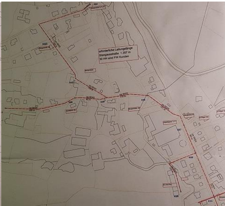
Erdgasnetz Stangau
